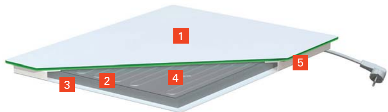
Schnittbild Vitoplanar Infrarotheizung
